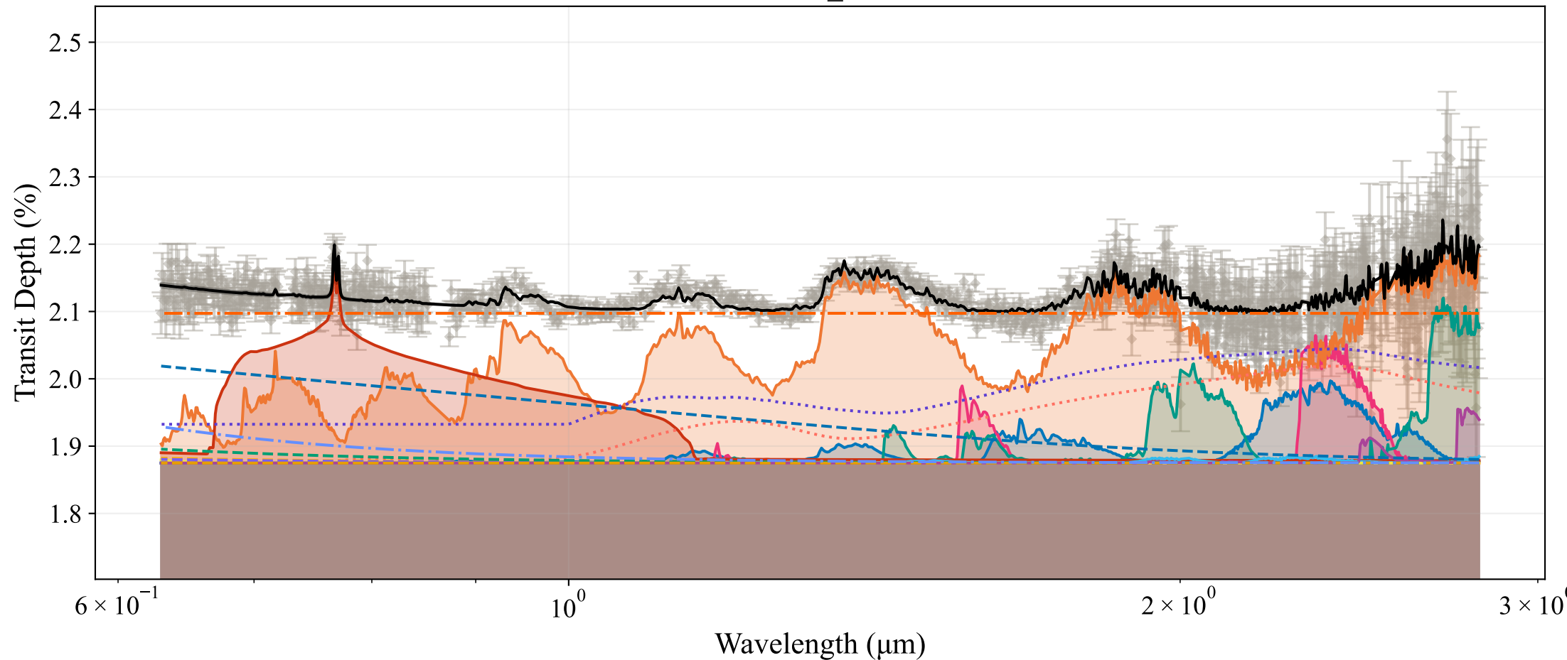
niriss_iso
